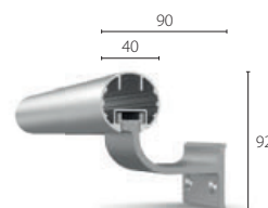
HRA-6-A60
