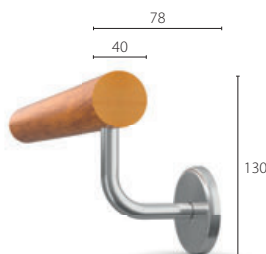
HRW-6-S75
