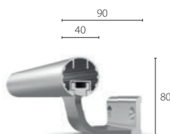
HRA-6-A80
